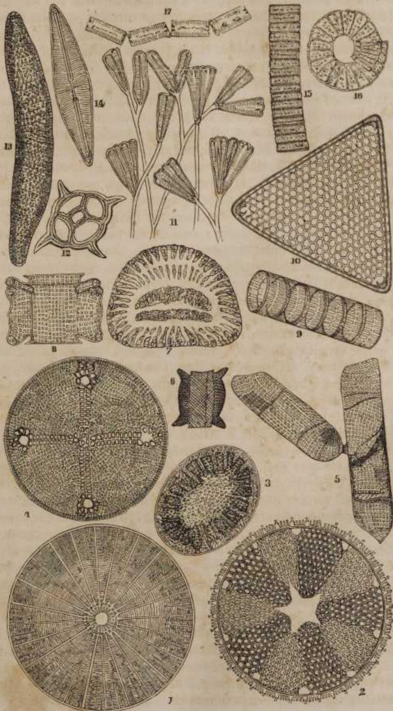
Fig.-Taf. 7. Diatomeen. Abbildung 1-17.
