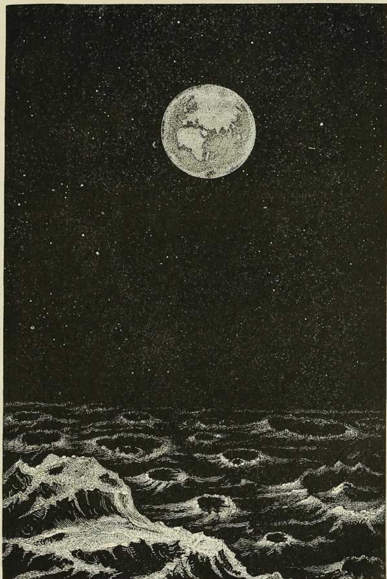
Die Erde, vom Monde aus gesehen.
