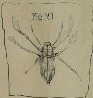
Fossiler Scorpion, vom Grafen Sternberg in einer böhmischen Kohlengrube gefunden (natürliche Grösse).
