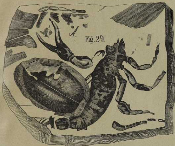
Fossiler Scorpion, vom Grafen Sternberg in einer böhmischen Kohlengrube gefunden (natürliche Grösse).
