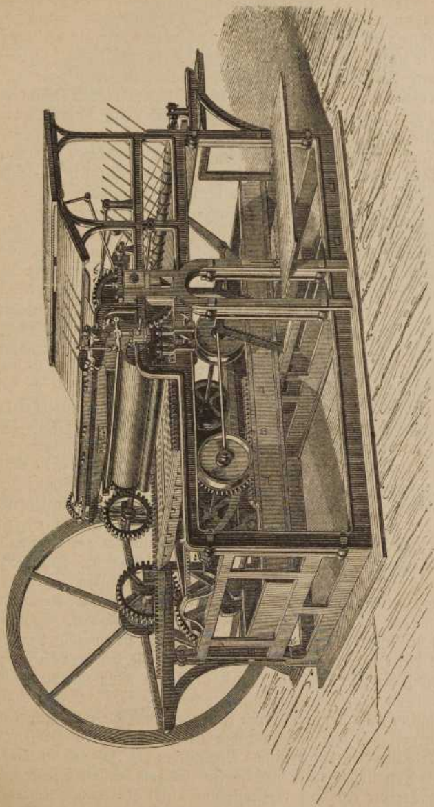
Einfache Schneltpresse mit Eisenbahnbewegung und Selbstausleger von König & Bauer.
