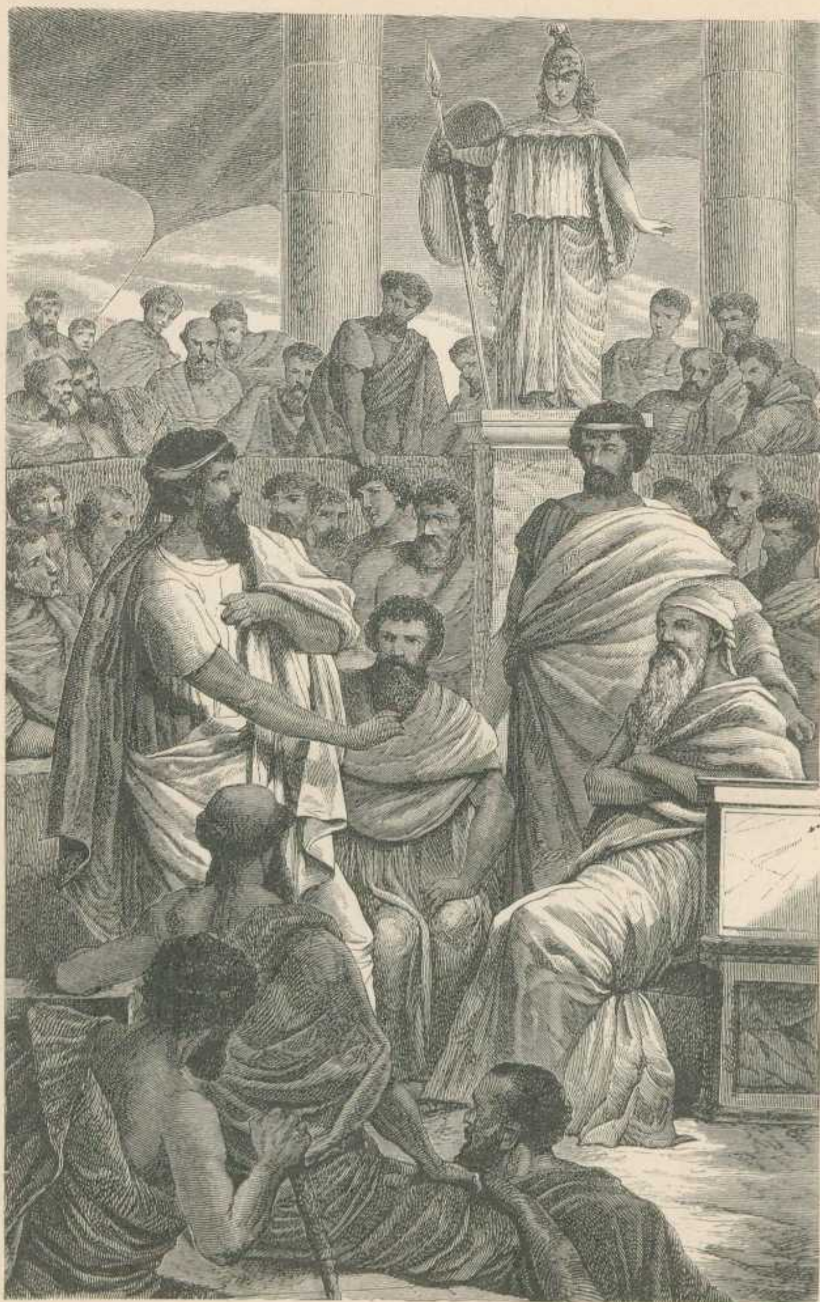
Pythagoras.
